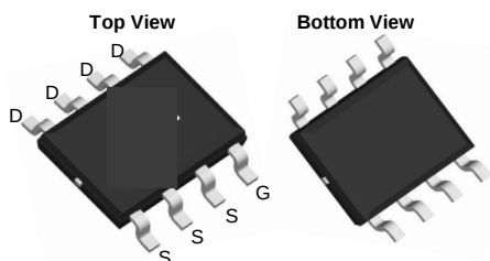
SOIC-8
